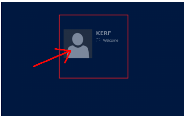
Figuur 9 – Aanmelden
